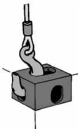
Пример захвата обычным крюком
