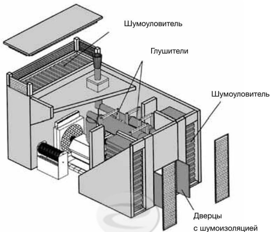
Пример установки
