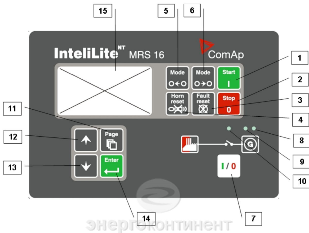
Кнопки управления генераторной установкой
